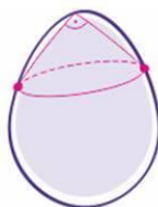
jajo Talesa
