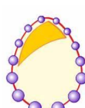
jajo Stewina
