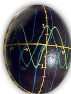
pisanka trygonometryczna
